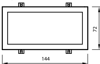
Dibujo de dimensiones A
